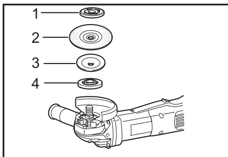
► 1. Contre-écrou 2. Meule flexible 3. Tampon d'ap- point 4. Bague interne
